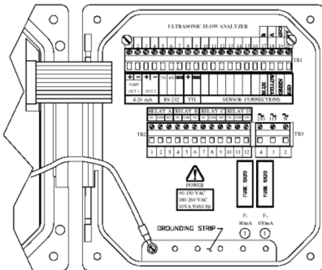
图 2-4 分析仪接线端子指示
