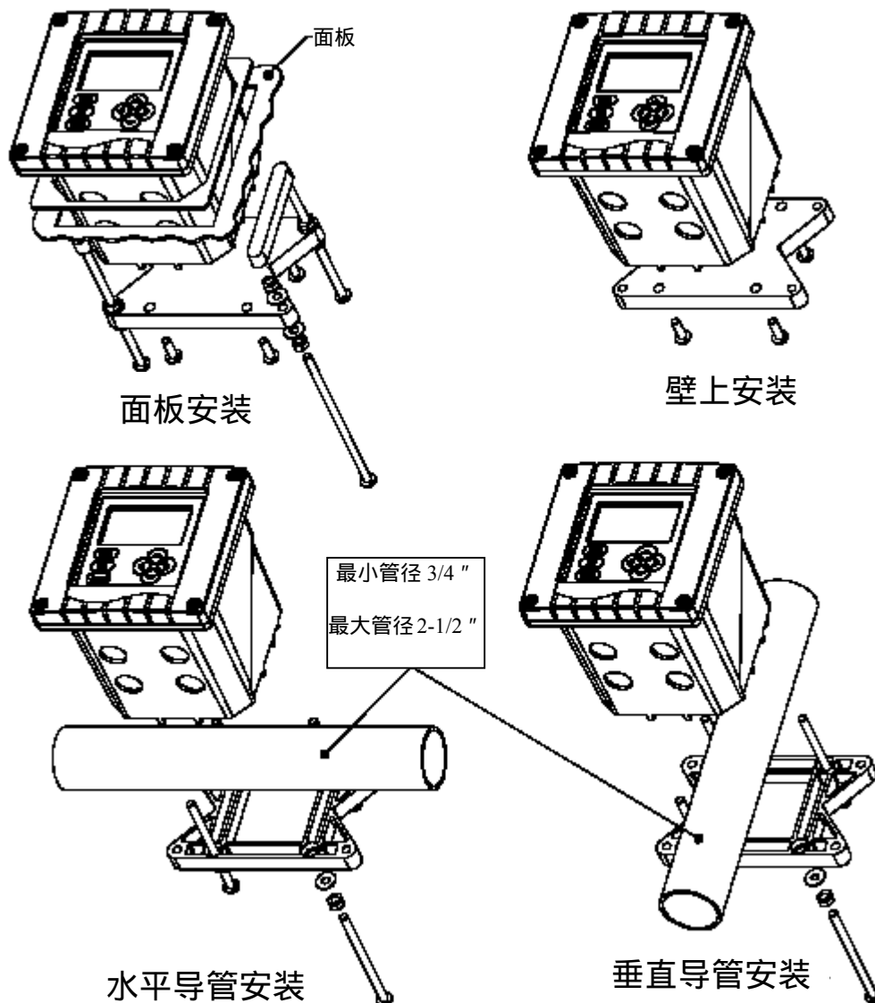
图 2-2 分析仪布置安装图
