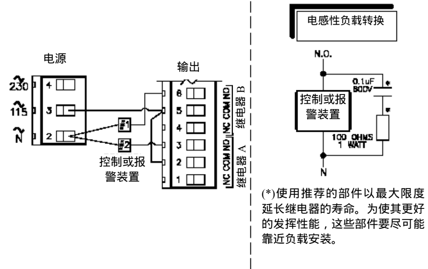
图 2-6 连接控制/报警装置与继电器
