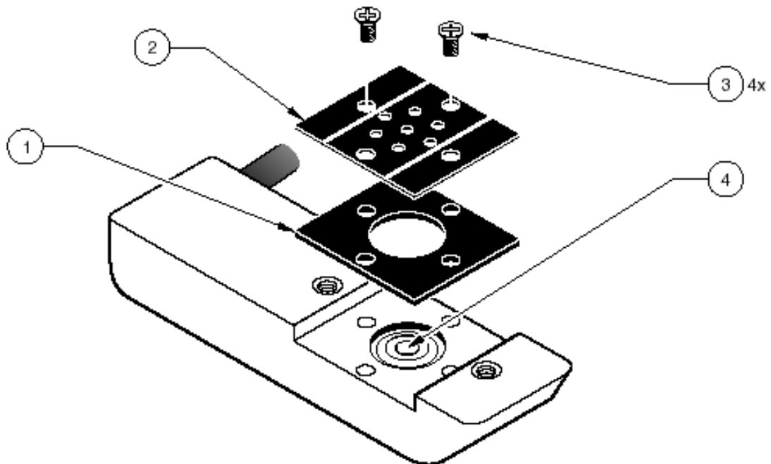
图 47 移开保护盖
